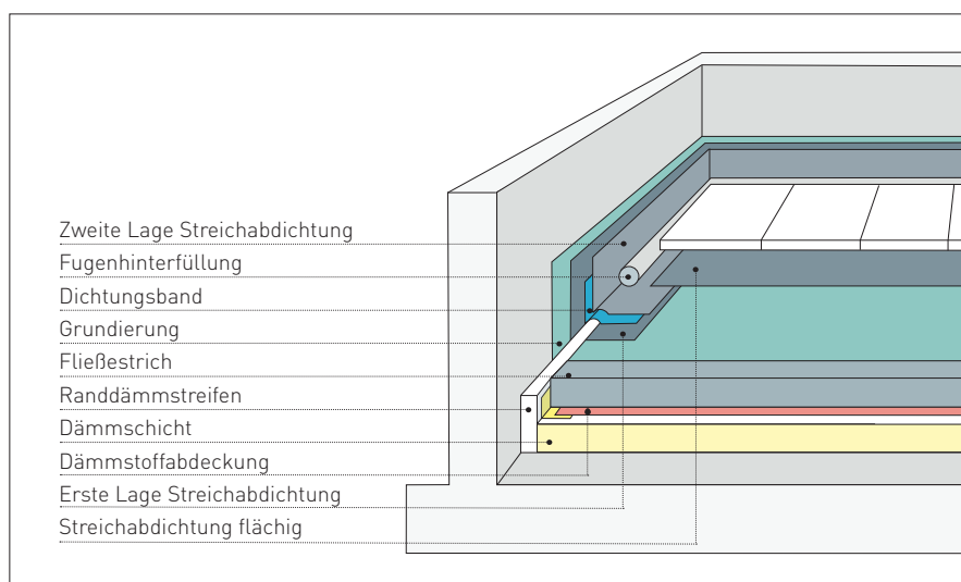
Streichabdichtung
